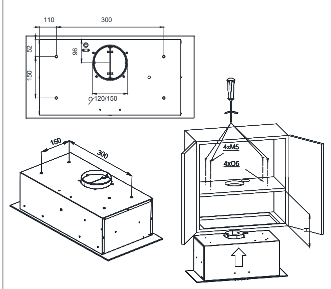
Obr. 6a: Montáž odsávača - horná montáž
