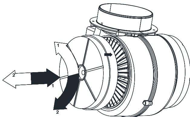
Obr. 7. Výmena uhlíkového filtra
