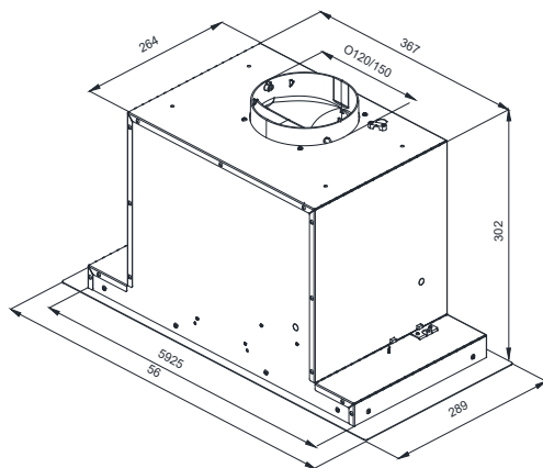
Obr. 2. Rozměry
