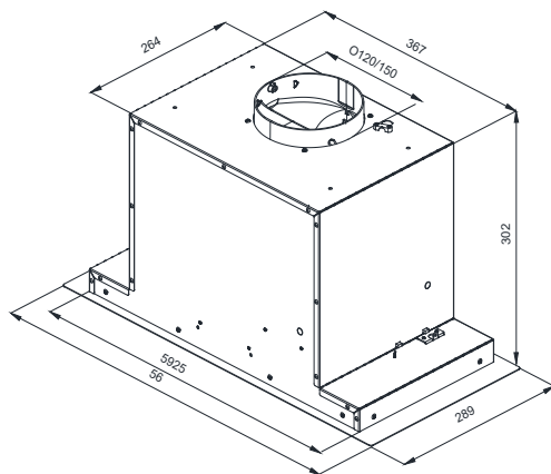
Obr. 2. Rozmery
