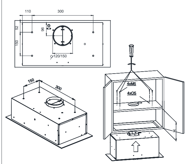
Obr. 6a: Montáž odsavače - horní montáž
