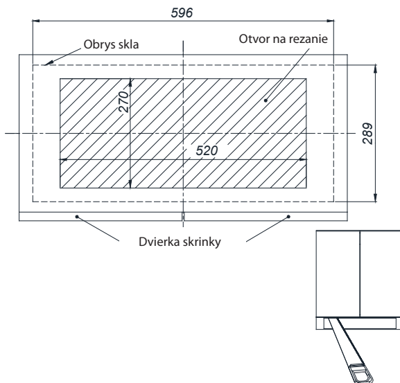
Obr. 4: Príprava skrinky
