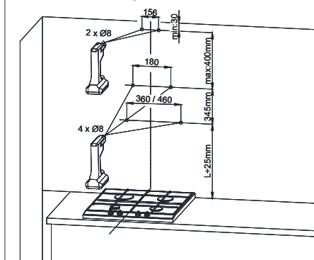
Obr. 6: Zavesenie odsávača pá
