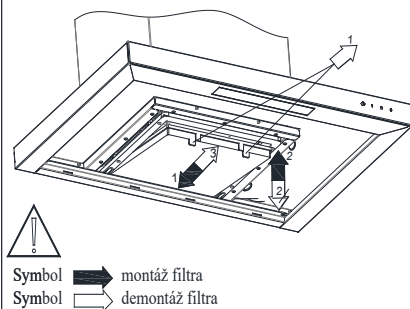
Obr. 10: Výmena filtra
