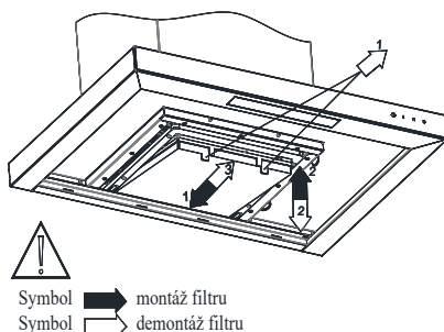
Obr. 10: Výměna filtru
