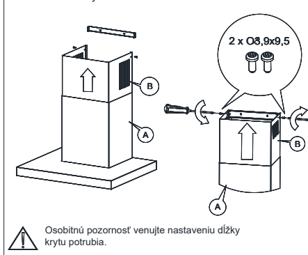
Obr. 9: Montáž krytu
