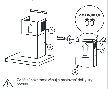
Obr. 9: Montáž krytu
