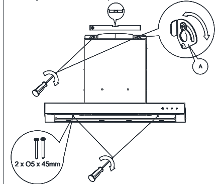
Obr. 8: Vyrovnanie odsávača pá
